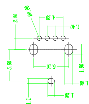
PCB LAY-UT (B-T-M VIEW)
